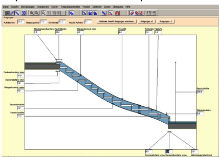
impresion de una escalera tipo cuarto caracol
