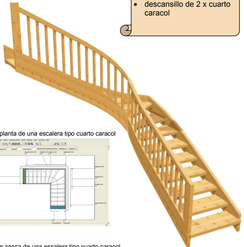
vista de zanca de una escalera tipo cuarto caracol
