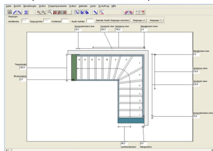
vista en planta de una escalera tipo cuarto caracol
